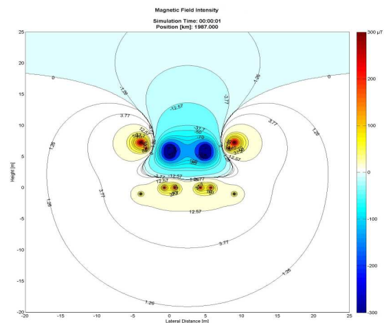
Intensidad de los campos magnéticos en una sección transversal de la línea de ferrocarril para una determinada posición y momento temporal
